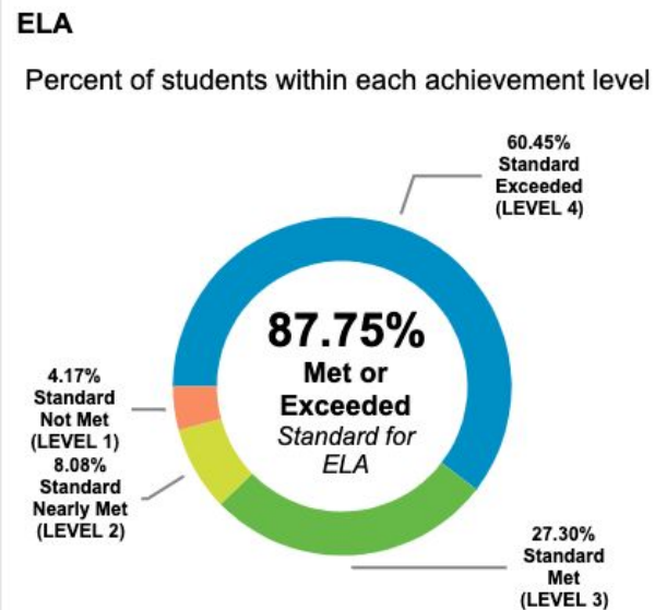
2017-18 ELA Scores
